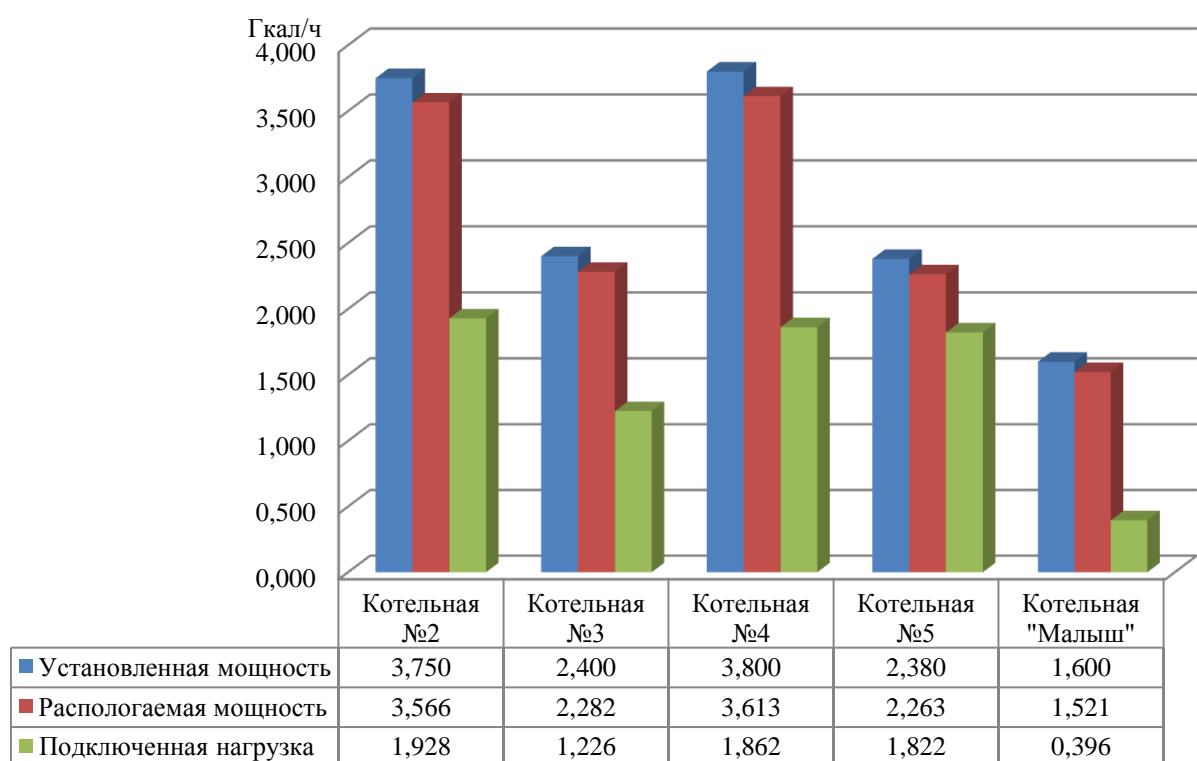
Рисунок 1.1 – Распределение мощностей источников тепловой энергии
